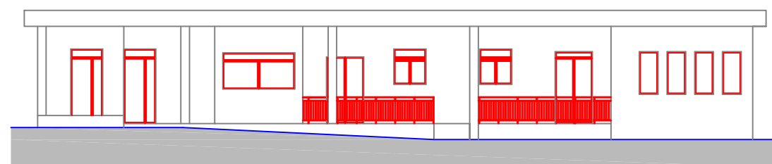
PROSPETTO SUD 1:200
